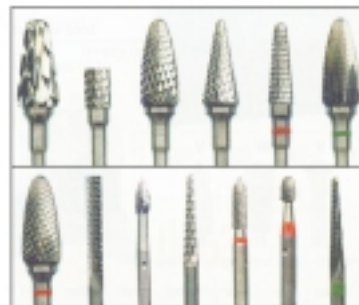
TUNGSTEN CARBIDE BURS
